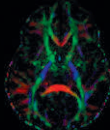
FA
